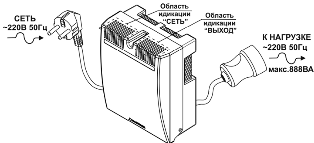
Рисунок 1 Внешний вид стабилизатора
