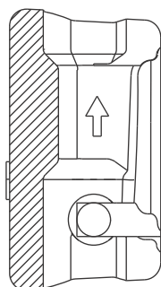
Рис. 19 Вид в разрезе, изолирующие оболочки
