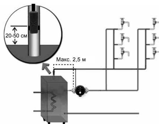
Рис. 7 Насос COMFORT BA PM, BXA PM со встроенным датчиком температуры
