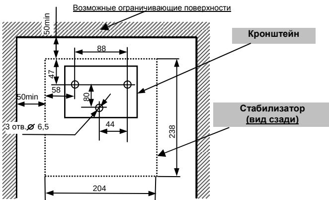
Рисунок 6.1 Схема размещения стабилизатора на стене
