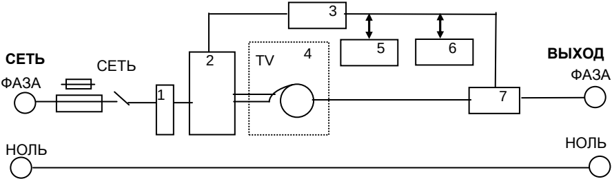
Рисунок 4.2 Структурно-функциональная схема изделия
