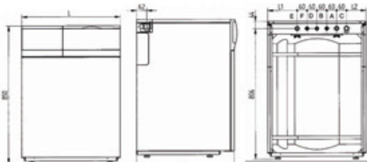
UB INOX 80 - 120 / SLIM UB INOX 80 - 120
