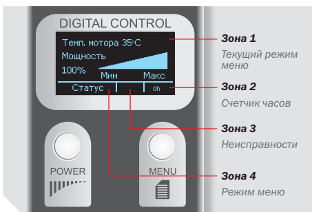
11. Дисплей электронного ассистента
