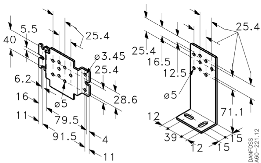
стенной кронштейн
