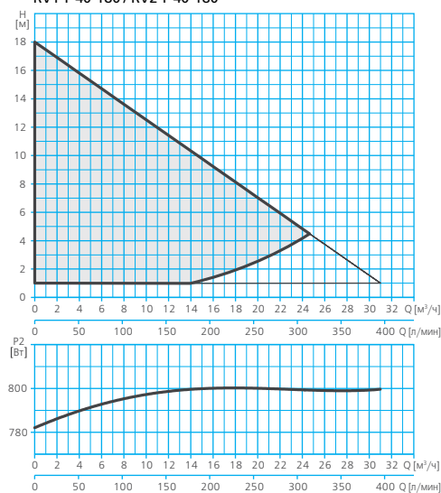
RV1-F 40-180 / RV2-F 40-180
