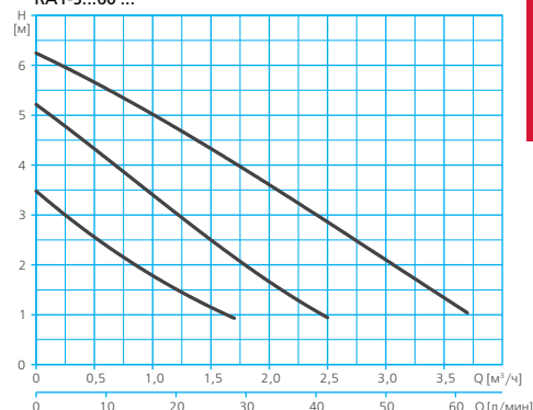
RA1-S...60 ...
