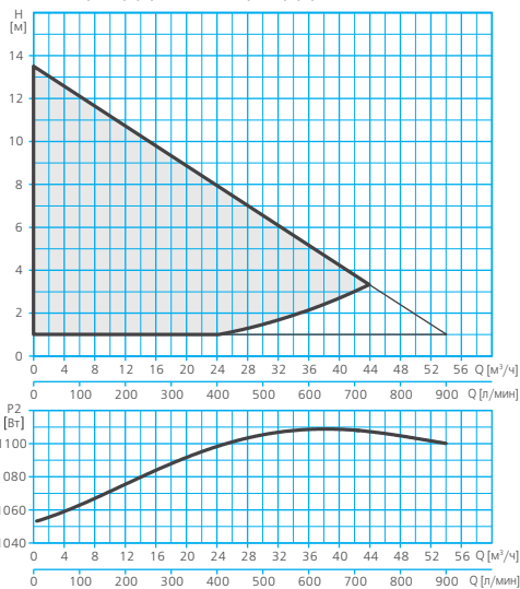
RV1-F (SAN) (X) 65 / RV2-F (SAN) (X) 65
