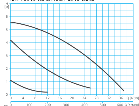
RA1-F 65-70 400 50 / RA2-F 65-70 400 50
