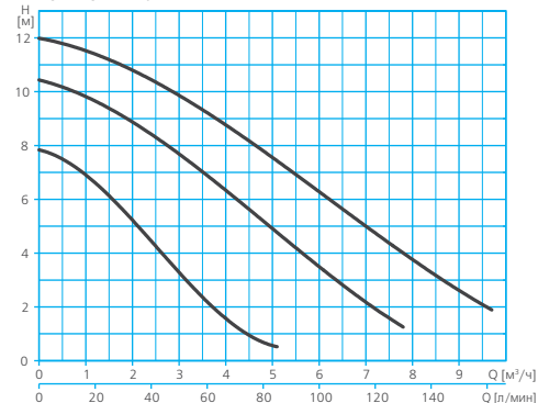
RSAN-5....-120 ...
