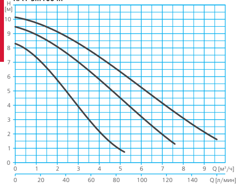
RA1-S...100 ...
