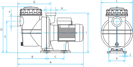
РАЗМЕРЫ И ВЕС
