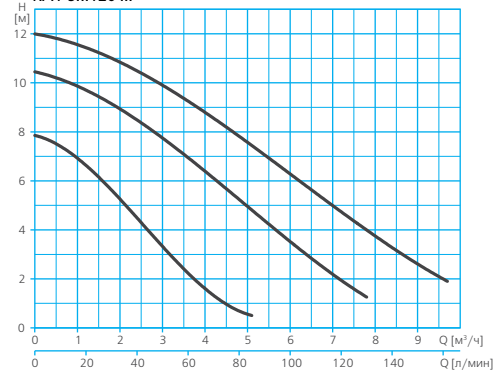
RA1-S...120 ...
