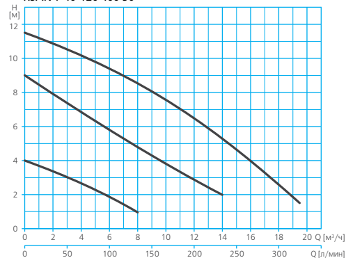
RSAN-F 40-120 400 50
