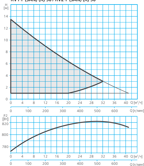
RV1-F (SAN) (X) 50 / RV2-F (SAN) (X) 50
