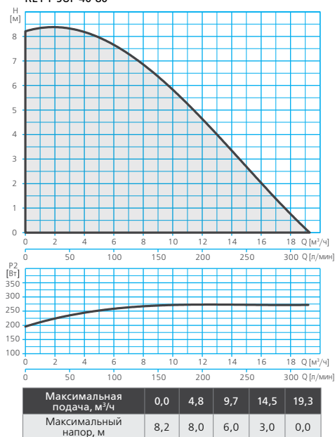
RE1-F SUP 40-80
