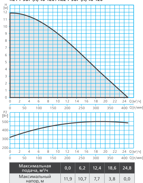
RE1-F SUP (X) 40-120 / RE2-F SUP (X) 40-120
