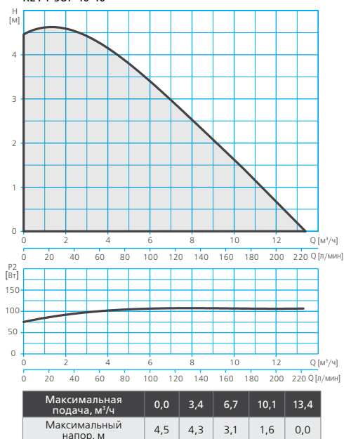
RE1-F SUP 40-40
