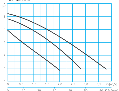
RA1-S...50 ...
