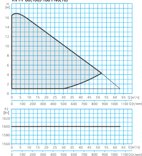
RV1-F 80(100)-180 PN6(10)
