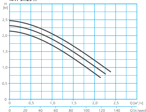
RA1-S...25 ...
