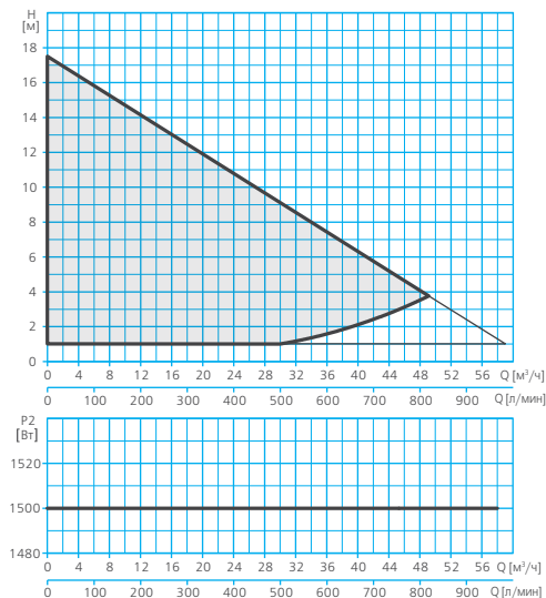
RV1-F 65-180 / RV2-F 65-180
