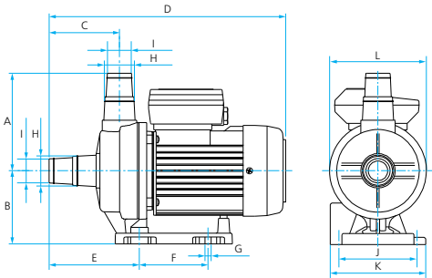
РАЗМЕРЫ И ВЕС
