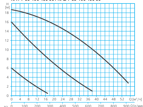
RA1-F 65-190 400 50 / RA2-F 65-190 400 50
