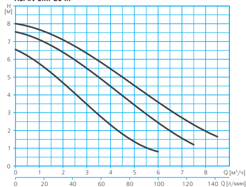
RSAN-S.....-80 ...
