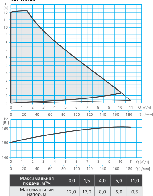
RE1-S...120
