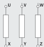
Соединение Треугольник-Звезда
