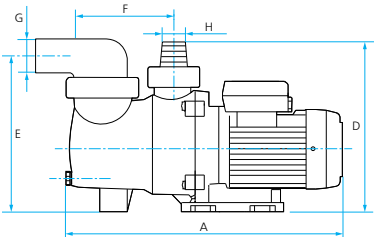
РАЗМЕРЫ И ВЕС
