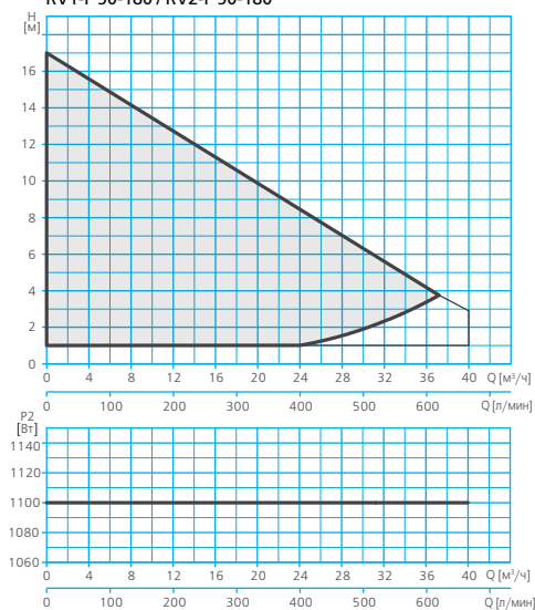
RV1-F 50-180 / RV2-F 50-180
