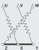
Схема соединений
