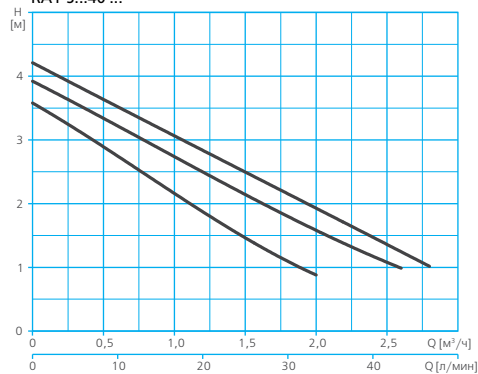
RA1-S...40 ...
