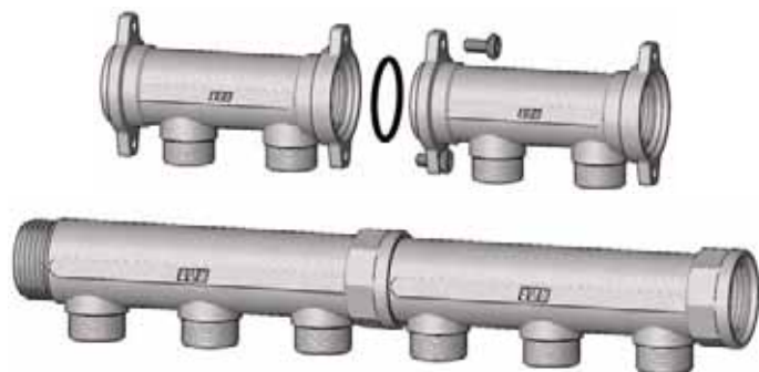
Рис. 3. Соединения коллекторов
