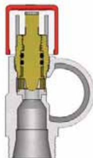
Рис. 20. Запорно-балансирующий коллектор
