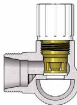
Рис. 13. Клапан запорно-балансирующего коллектора
