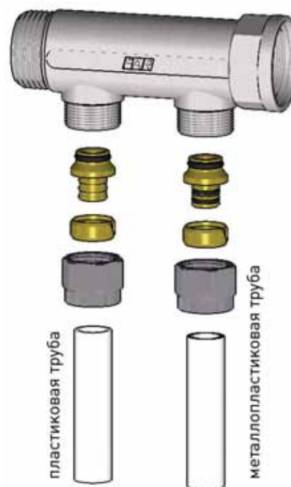
Рис. 38. Присоединение к отводам eurokopus
