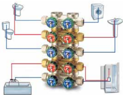
Рис. 5. Подключение регулируемого параллельного коллектора
