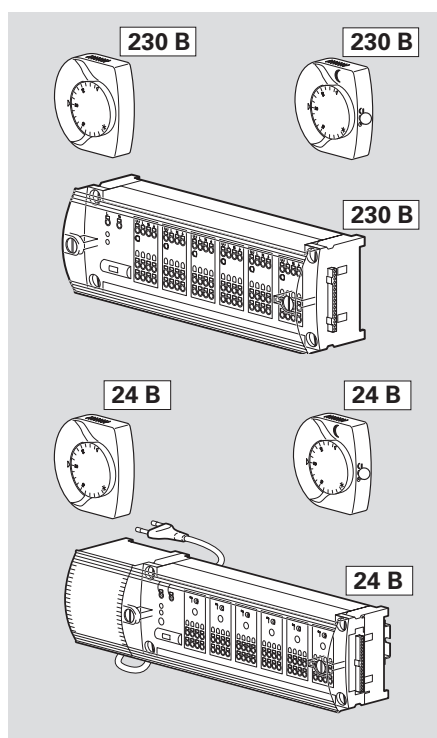
Рис. 5 Клеммная колодка и комнатные термостаты
