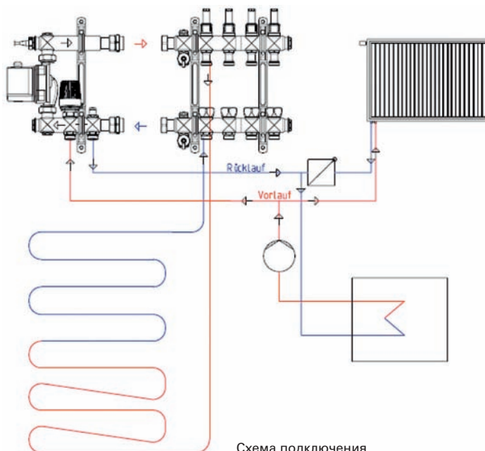
Схема подключения
