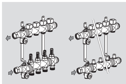
Рис. 4 Распределительный коллектор
