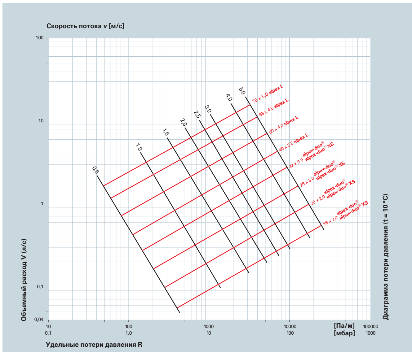
Диаграмма потерь давления в трубопроводах питьевого водоснабжения ( \vartheta_m = 60\text{ }^\circ\text{C} )
