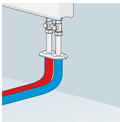
Отдельное присоединение к распределителю alrex (лучевая разводка)
