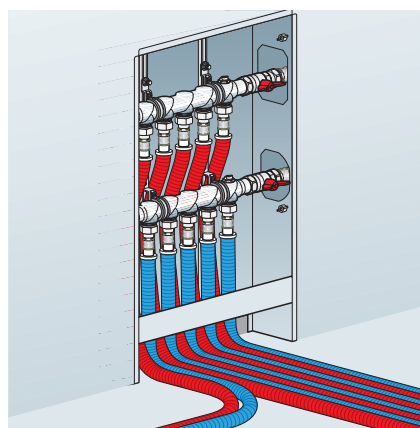
Монтаж коллектора в специальном распределительном шкафу
