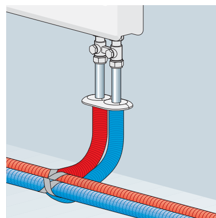
Подключение тройниками alrex
