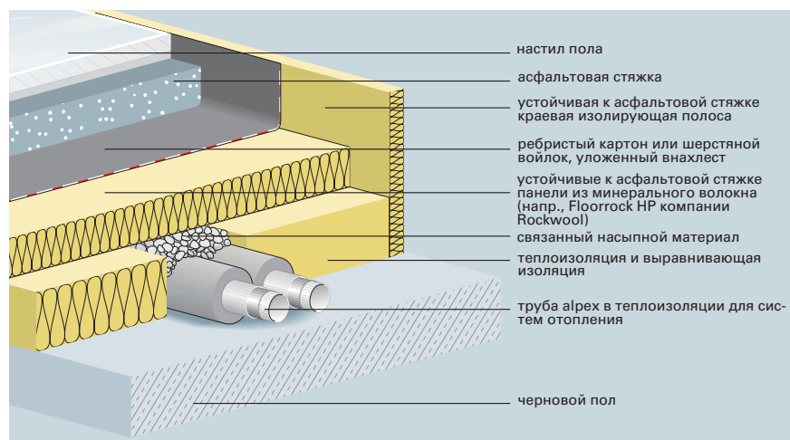
Конструкция пола под асфальтовой стяжкой
