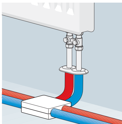
Присоединение с помощью перекрестного сдвоенного тройника alrex-duo
