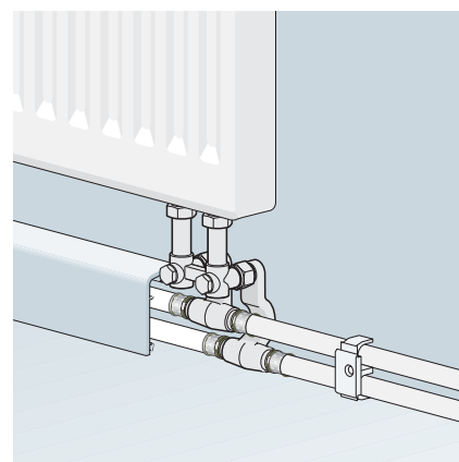
Плинтусное подключение alrex-duo®
