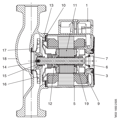
Рис. 17. Трехфазный насос UP
