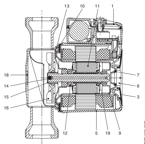
Рис. 16. Однофазный насос UP, насос типа SOLAR
