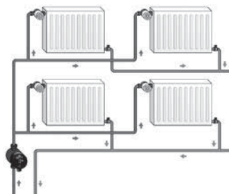
Рис. 7. Двухтрубная система отопления
