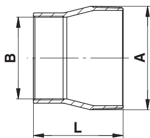
Рис. 31 Габаритный чертеж и изображение соединительной детали резьба-резьба
