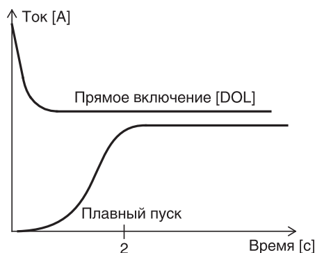
Рис 6. Сравнение пусковых токов.
