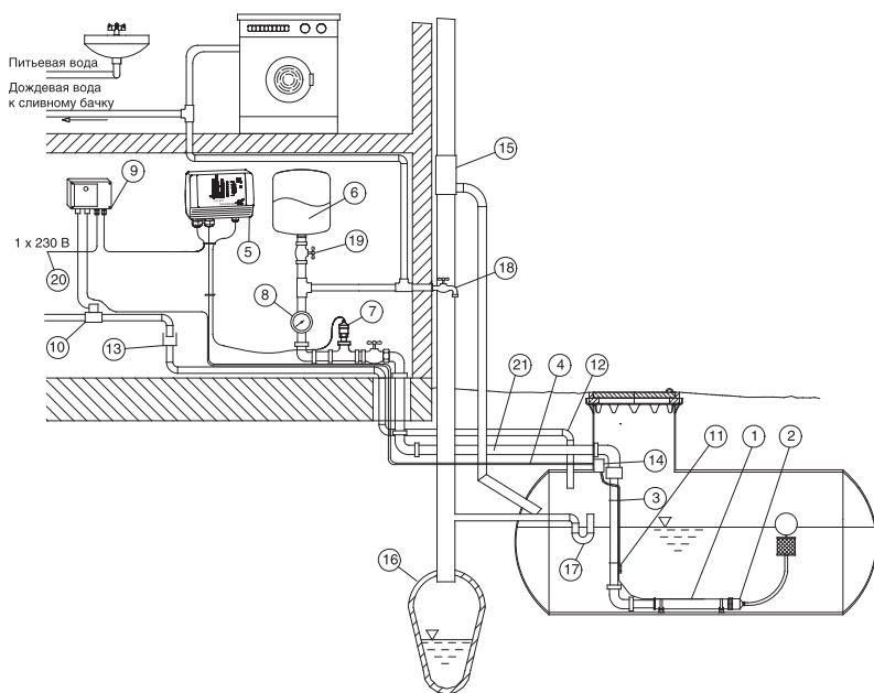
Рис 17. Насос типа SQE в системе альтернативного использования дождевой воды.
