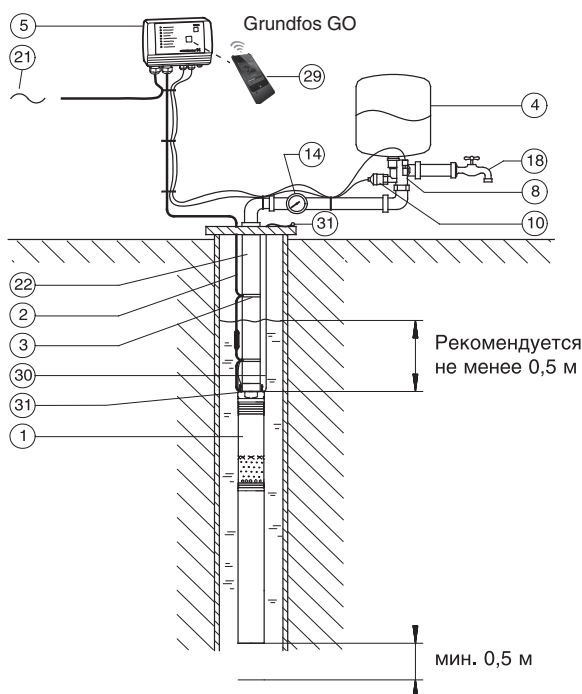
Рис 13. Насос типа SQE и CU 300 в системе водоснабжения (поддержание постоянного давления).
