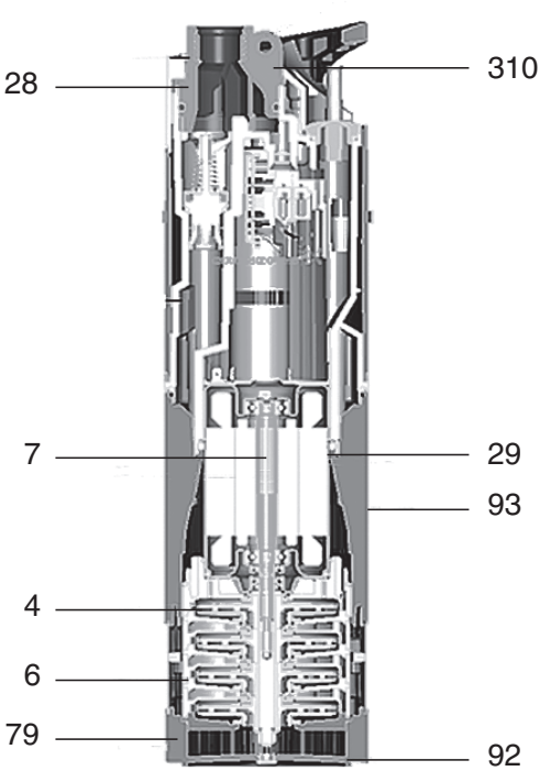
Рис. 42. Разрез установки SBA
