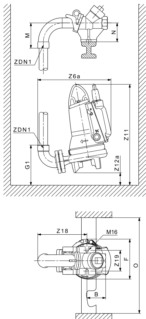
Рис. 24 Установка на надводной автоматической трубной муфте
