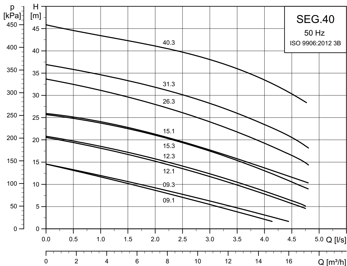
Рис. 4 Рабочий диапазон
