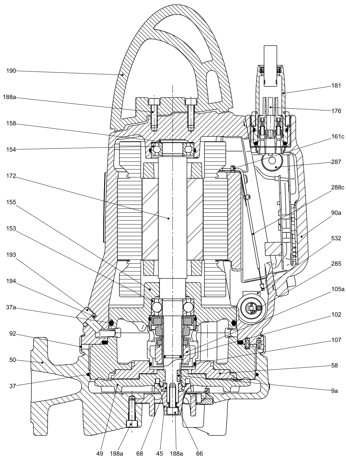
Рис. 11 Чертеж насоса SEG AUTO ADAPT в разрезе, 2,6, 3,1 и 4,0 кВт
