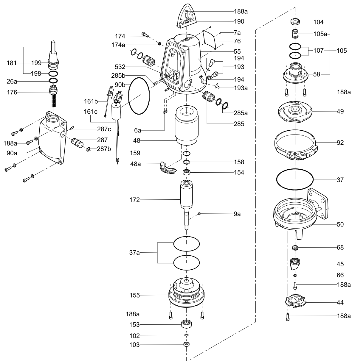
Рис. 10 Детализовка насоса SEG AUTO ADAPT , 0,9, 1,2 и 1,5 кВт
