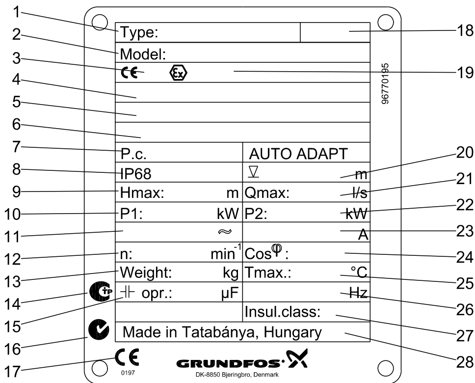
Рис. 3 Фирменная табличка на насос SEG AUTO ADAPT
