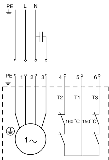
Рис. 16 Схема соединений для насосов SEG с однофазными электродвигателями. Смотрите таблицу ниже
