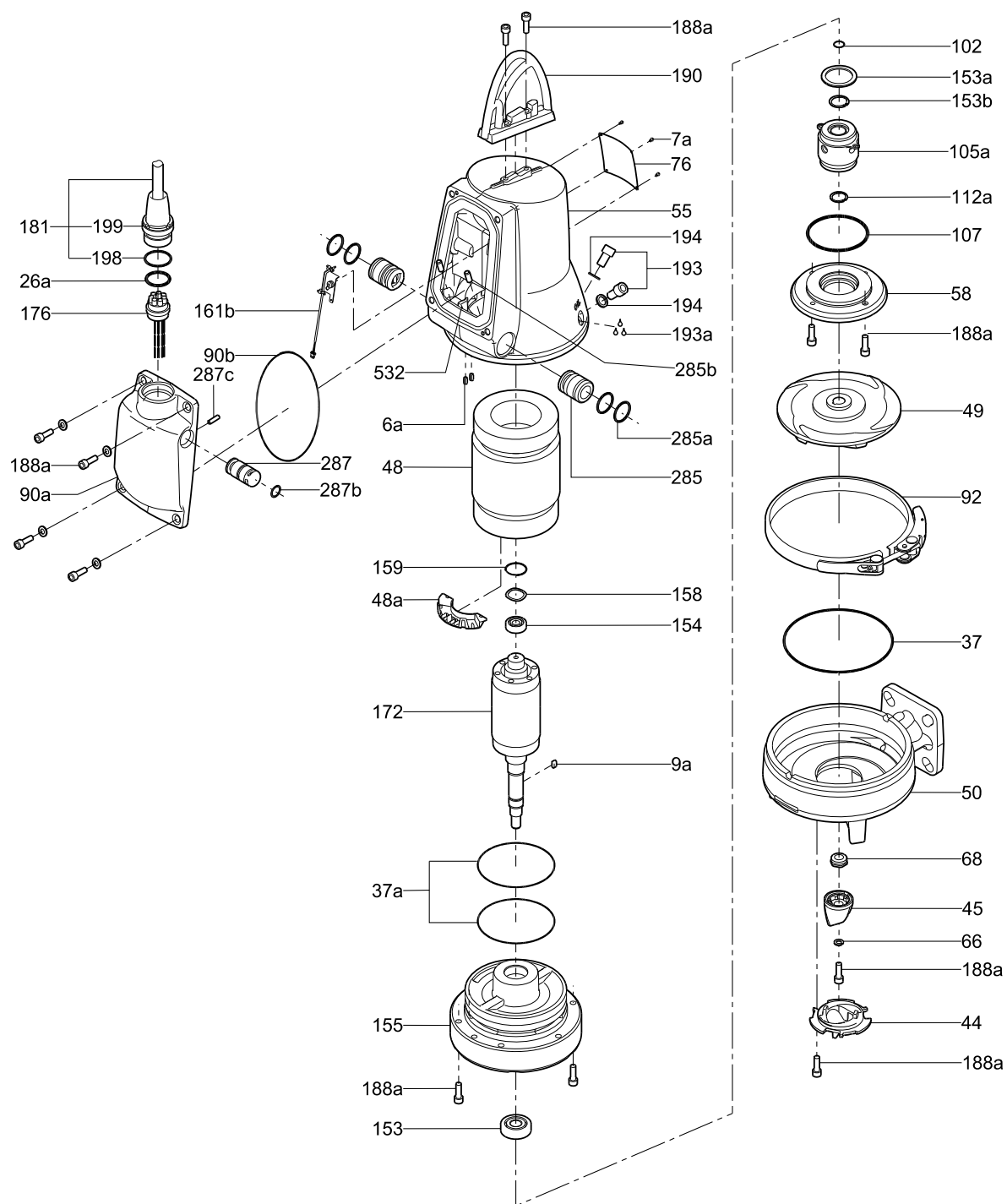
Рис. 12 Детализовка насоса AUTO ADAPT , 2,6, 3,1 и 4,0 кВт
