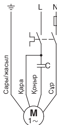
22-сур. Franklin фирмасының электр қозғалтқыштары
