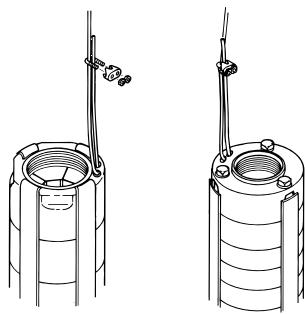
Рис. 15 Закрепление страховочного троса
