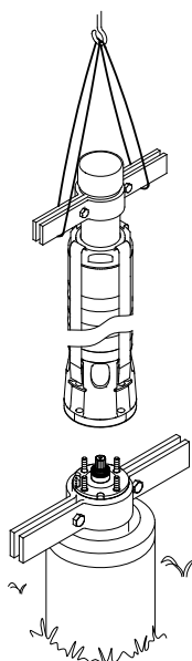
14-сур. Сорғыны көтеру жәнке орнату
