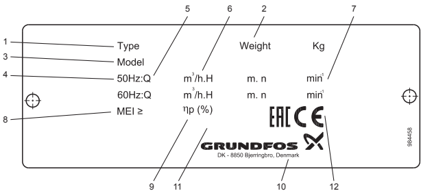
Рис. 3 Фирменная табличка насосов SP(SPM) 1A...14 и SP(SPM) 77...215
