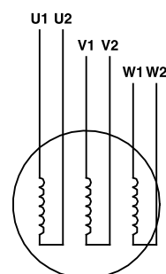
26-сур. Кабель/клеммалардың белгісіз таңбалануы - «Жұлдыз-үшбұрыш» сызбасы бойынша іске қосуға арналған электр қозғалтқыштарының орамы
