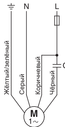
Рис. 21 Электродвигатели PSC
