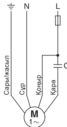
21-сур. PSC электр қозғалтқыштары
