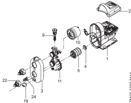
Рис. 2 Конструкция SCALA2
