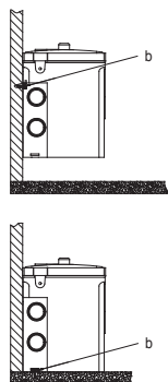
Рис. 4 Пример монтажа резервуара на стене и на полу
