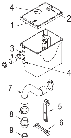
1-сур. Liftaway C сұйыққоймасының жиынтығы
