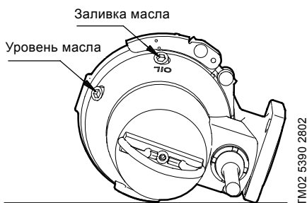
Рис. 13 Отверстия для заливки масла
