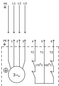
Рис. 5 Схема соединений для насосов с трёхфазными электродвигателями
