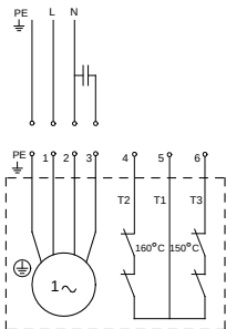
Рис. 4 Схема соединений для насосов с однофазными электродвигателями
