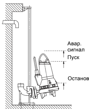
Рис. 6 Уровни пуска и останов насоса
