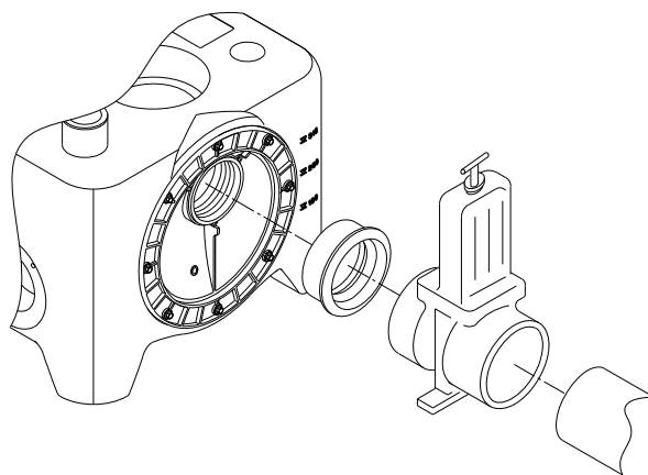
Рис. 21 Монтаж задвижки
