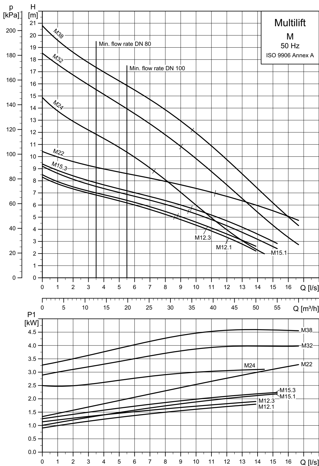
Рис. 34 Рабочие характеристики
