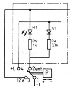
Schaltbild
