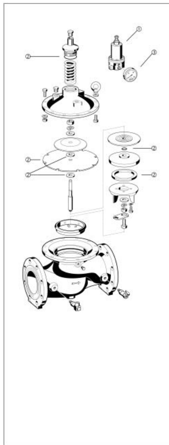
Запасные части для редукционных клапанов DR 300 (начиная с 2002 г.)
