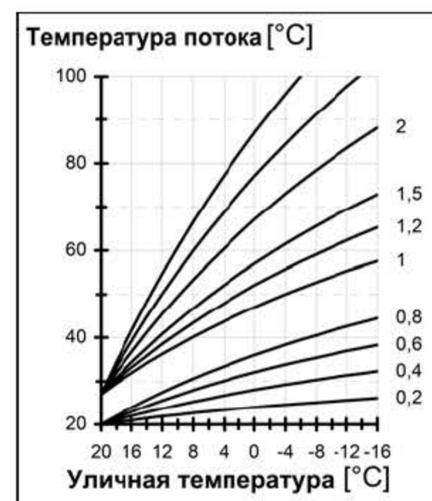
Диаграмма кривых отопления
