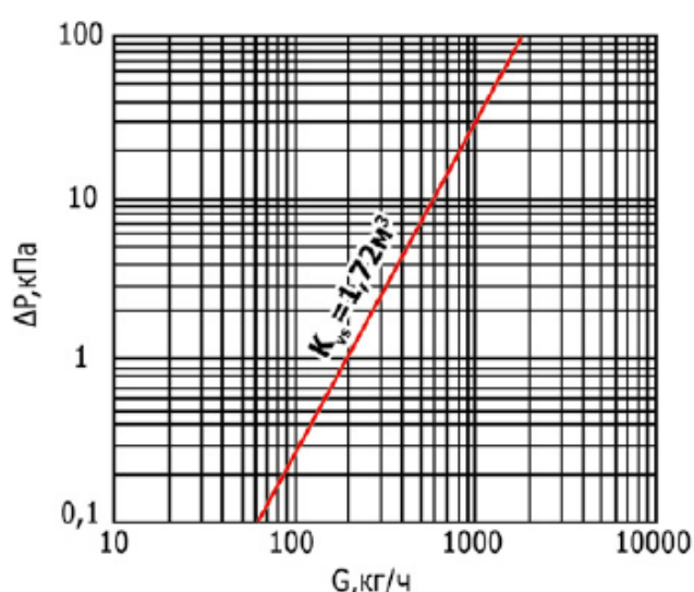
Диаграмма клапана ручного терморегулирующего SVR DN 20 прямого
