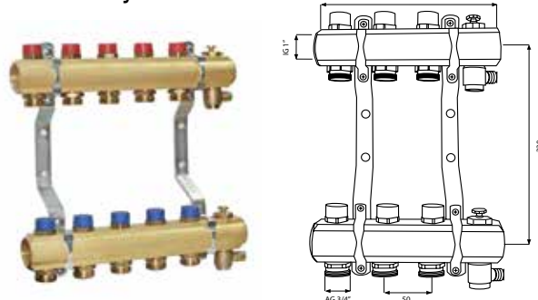
Латунь
