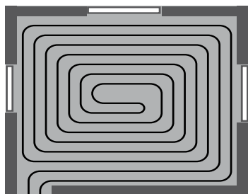
Укладка трубопровода в форме улитки
