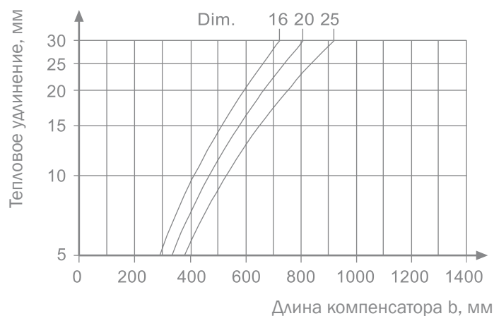
Температурный компенсатор для универсальных труб TECElogo
