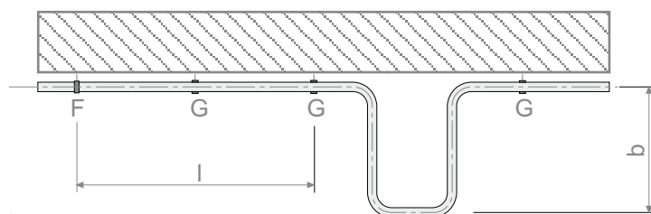
b - длина компенсатора, мм; l - длина трубопровода, м; F - неподвижная опора; G - скользящая опора.
