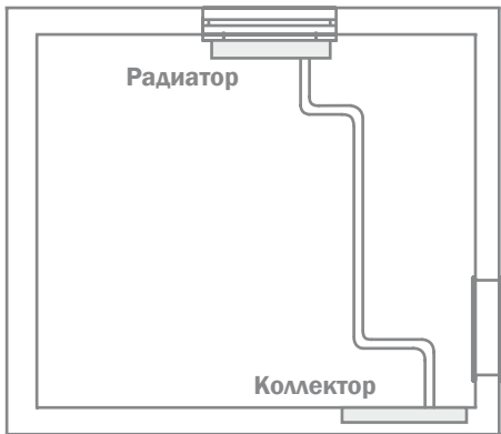
Пример прокладки трубы с учетом термического удлинения
