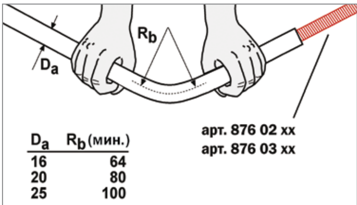
Изгибание трубы TECElogo с использованием пружины
