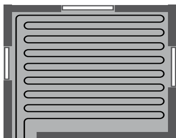
Укладка трубопровода в форме меандра
