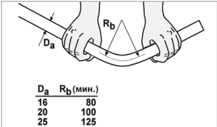
Изгибание трубы TECElogo без пружины
