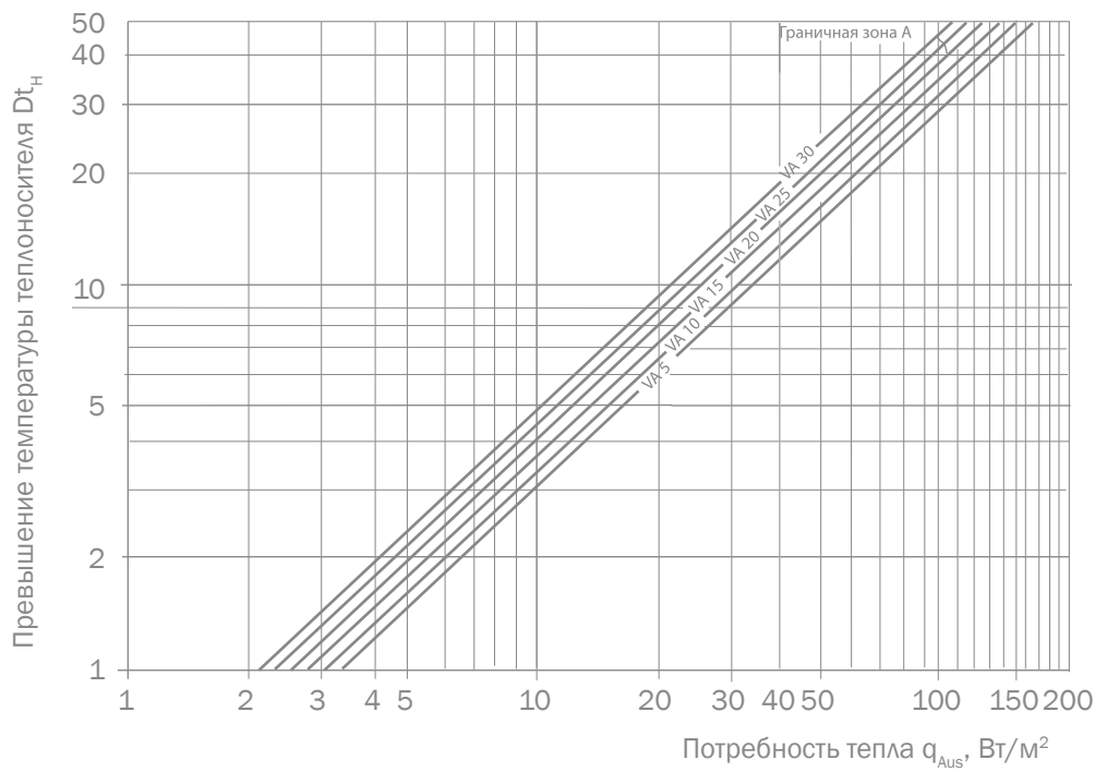
Диаграмма определения температуры поверхности пола. Покрытие пола: R\lambda=0,15 \text{ м}^2\text{Вт/К}
