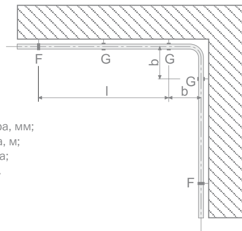
Пример оборудования компенсатора при смене направления трубопровода
