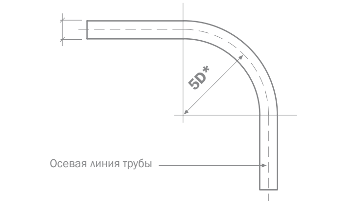
* Без изгибающей пружины и трубогиба (с пружиной или трубогибом 4 диаметра) Минимальный радиус изгиба труб TECElogo
