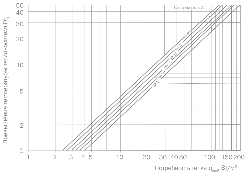
Диаграмма определения температуры поверхности пола. Покрытие пола: R\lambda=0,10 \text{ м}^2\text{Вт/К}
