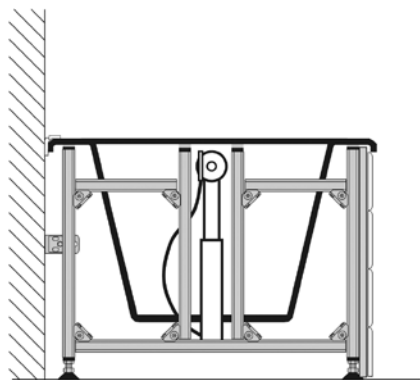
Несущая конструкция TЕСEprofil при монтаже сифона
