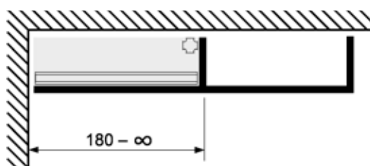
Сооруженная шахта
