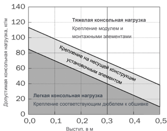
Консольные нагрузки
