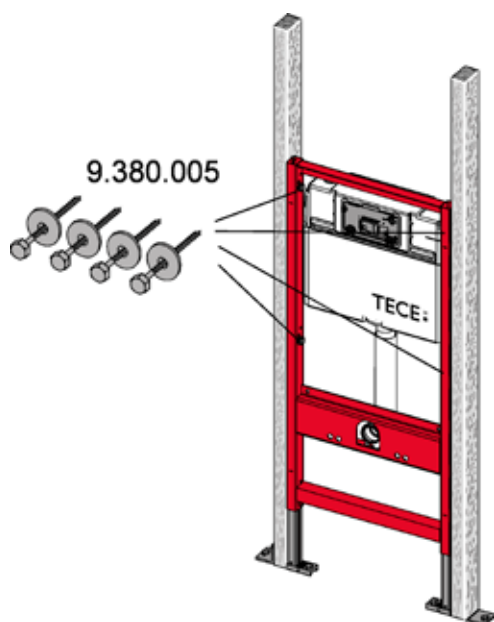
Крепление модуля при монтаже в стене с деревянным каркасом
