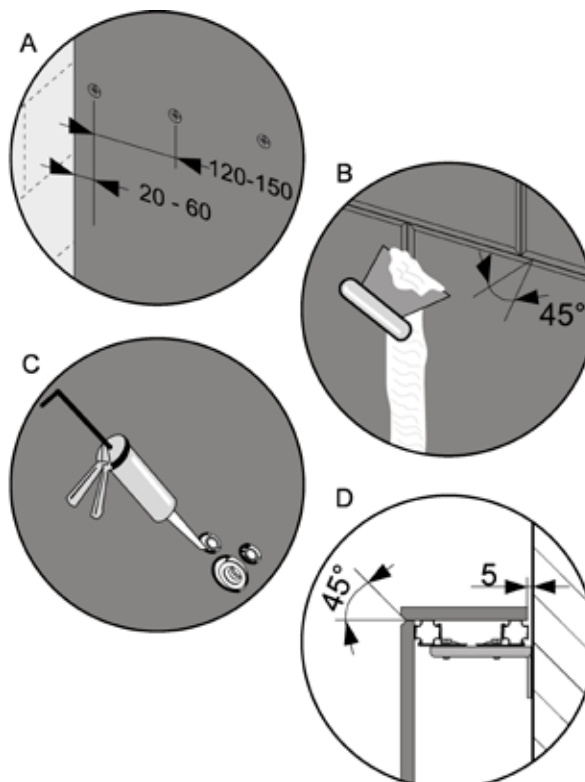
Обшивка несущей конструкции TЕСEprofil и нанесение шпаклевки
