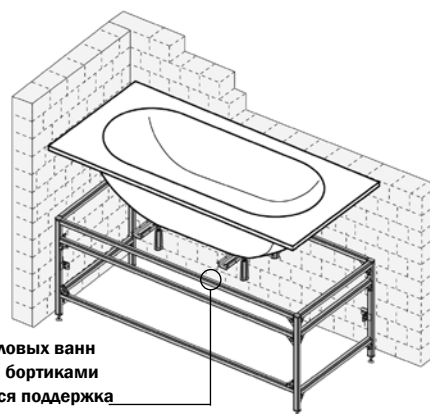
Монтаж опор для акриловой ванны
