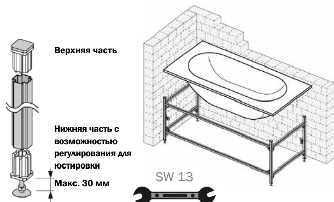
Установка стальной ванны в несущий каркас TECEprofil
