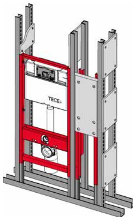
Монтаж модуля для поручней и опорных систем с UA-профилем в свободстоящей стене
