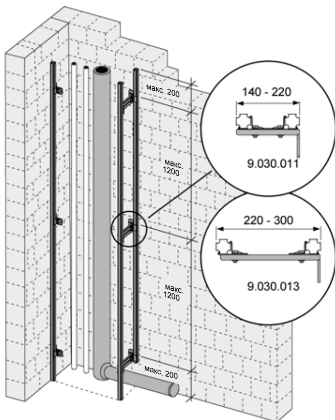
Сооруженная шахта
