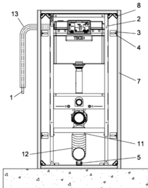
Опытная конструкция фальшстены TECEprofil с туалетным модулем
