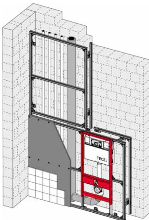
Сооруженная шахта
