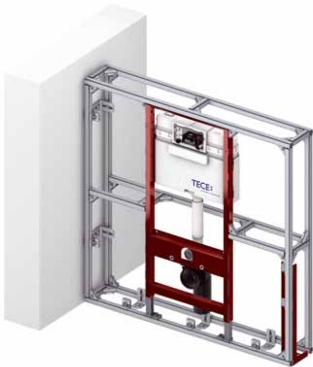
Монтаж в свободностоящую стену TECЕprofil
