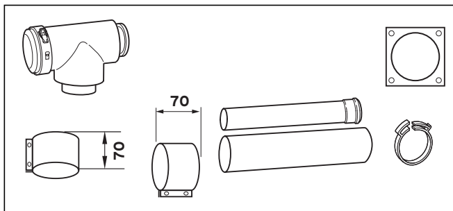
Рис. 4.18 Объем поставки
