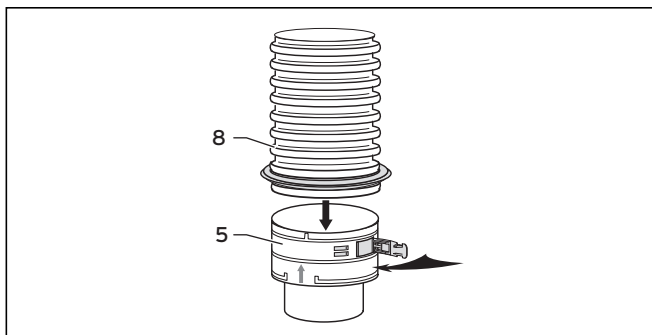
Рис. 4.39 Вставной элемент с гибким отводом ОГ
