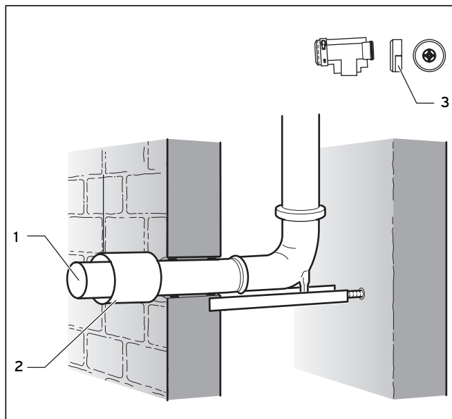
Рис. 4.27 Эксплуатация с забором воздуха из помещения (прямая установка)
