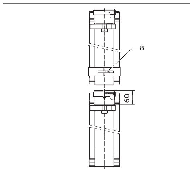
Рис. 4.72 Соединение компонентов ОГ на внешней стенесистемы
