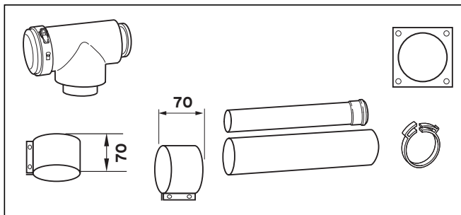
Рис. 4.15 Объем поставки
