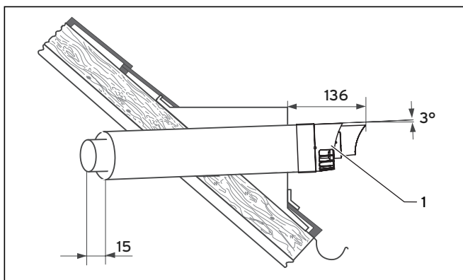
Рис. 4.11 Встройка горизонтального кровельного ввода
