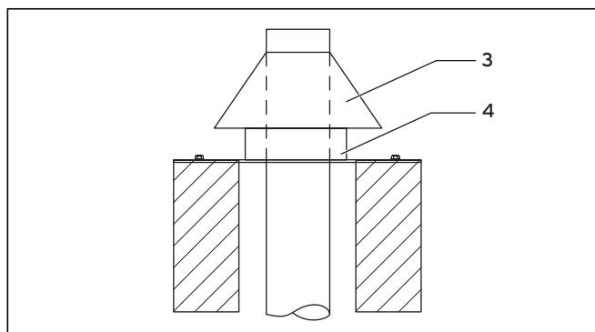
Рис. 4.50 Монтаж шахтного кожуха
