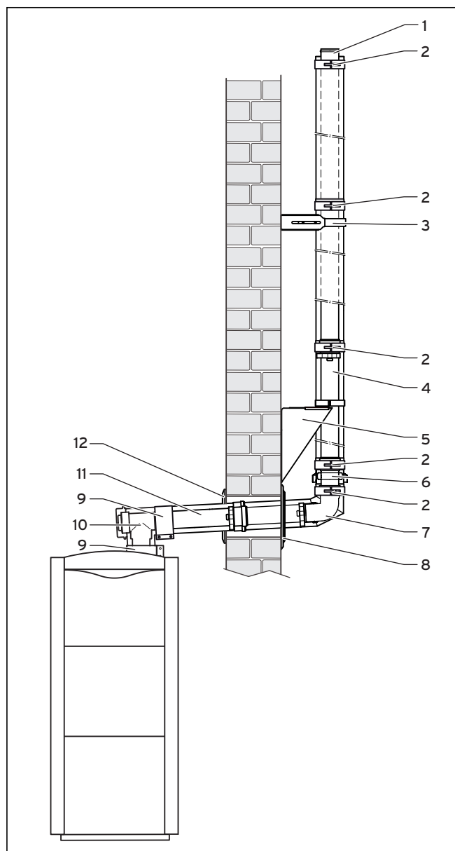
Рис. 4.67 Системное представление отвода ОГ
