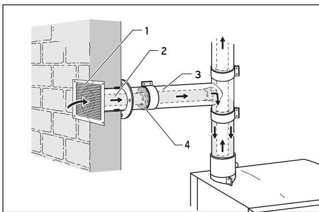
Рис. 4.30 Подвод воздуха через наружную стену
