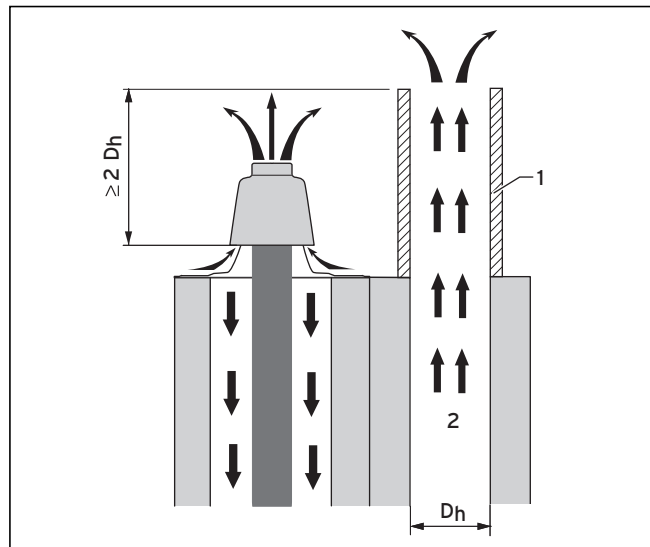
Рис. 4.45 Выпускной газопровод в шахте рядом с системой выпуска отработанных газов, которая не должна быть устойчивой к горению сажи
