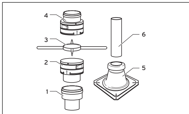
Рис. 4.53 Гибкий отвод ОГ, комплект 1
