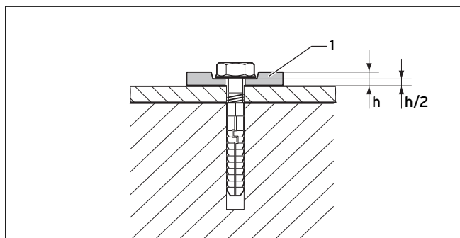
Рис. 4.42 Крепление гибкими подкладными шайбами
