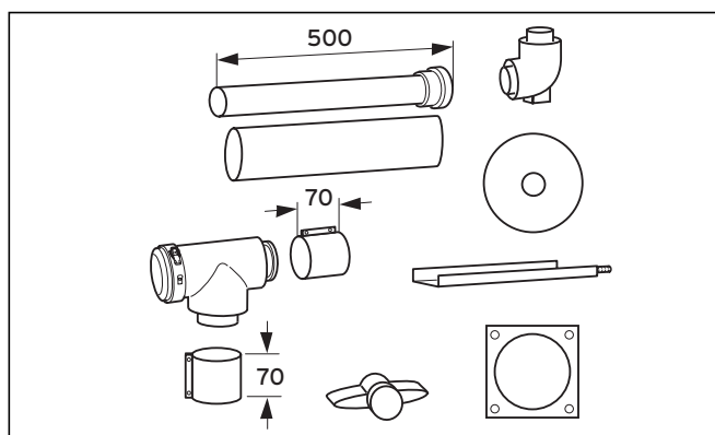
Рис. 4.79 Объем поставки
