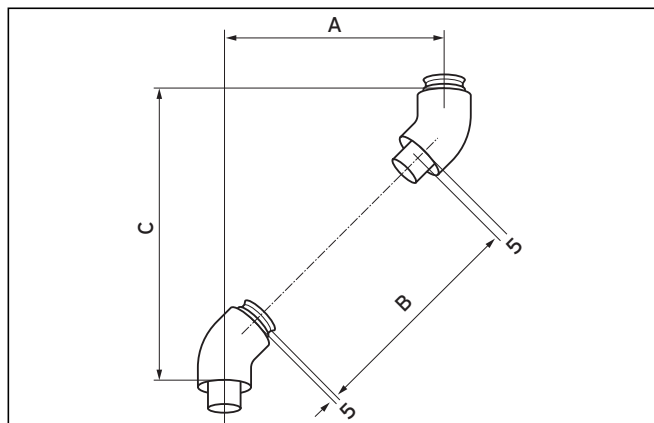
Рис. 4.89 Монтаж колен 45°
