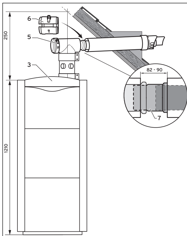
Рис. 4.13 Прямая установка
