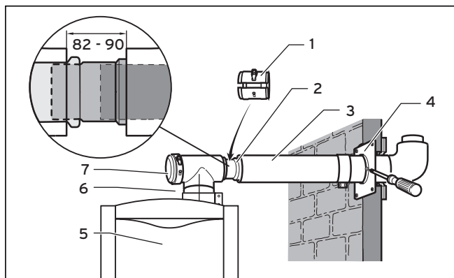
Рис. 4.78 Монтаж патрубка отвода ОГ
