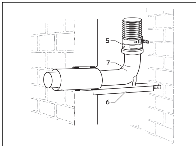
Рис. 4.41 Концентрическое подключение к гибкому отводу ОГ
