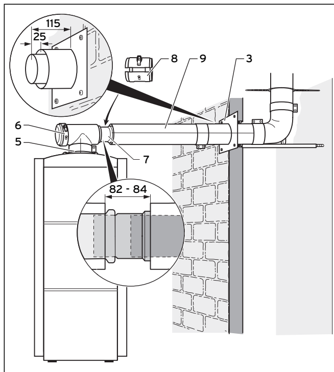
Рис. 4.85 Удаленная установка
