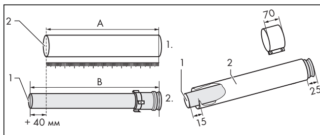
Рис. 4.87 Укорачивание труб
