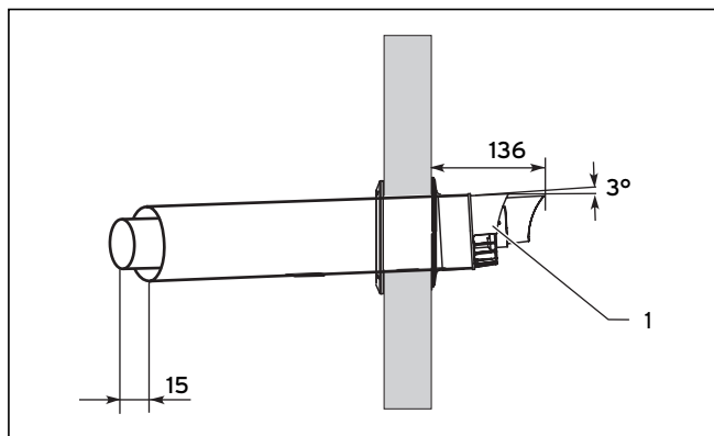
Рис. 4.12 Монтаж горизонтального вывода через стену
