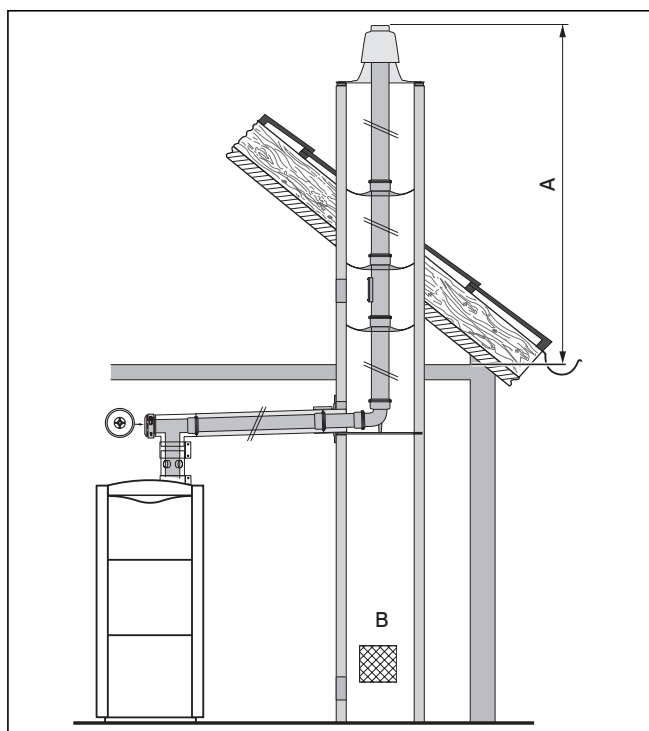
Рис. 4.23 Пример монтажа с забором воздуха из помещения
