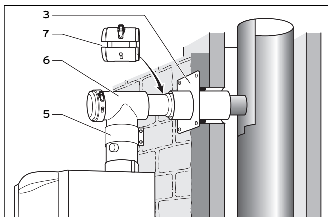
Рис. 4.17 Монтаж аппарата
