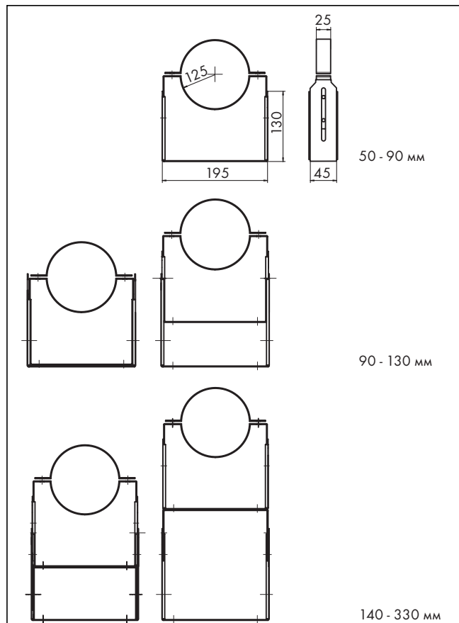
Рис. 4.74 Диапазон настройки кронштейнов на наружной стене
