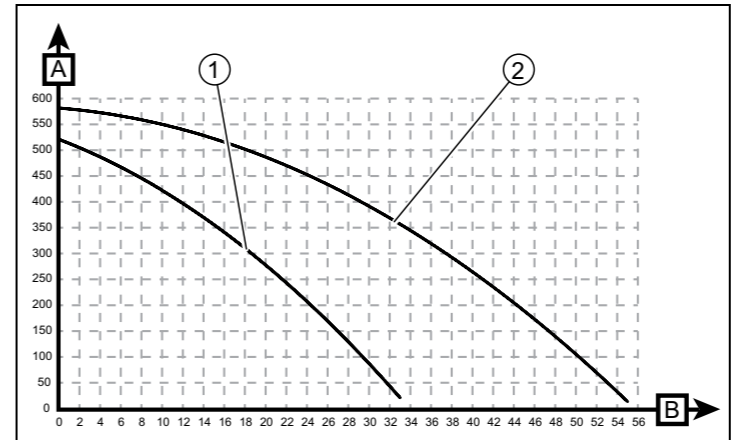
Характеристическая кривая циркуляционного насоса atmoTEC/turboTEC plus VU
