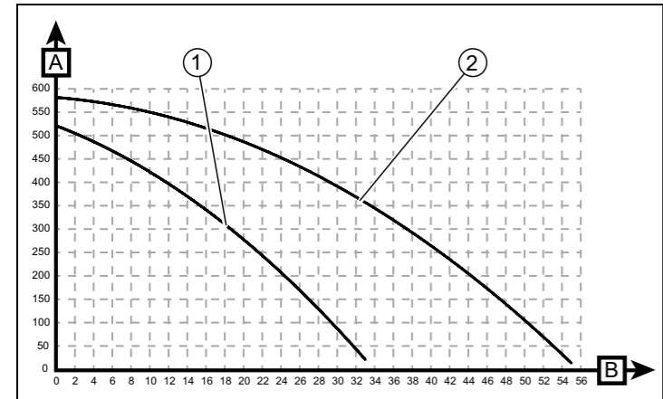
Характеристическая кривая циркуляционного насоса turboTEC pro VUW
