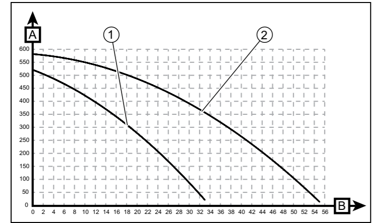
Характеристическая кривая циркуляционного насоса atmoTEC/turboTEC plus VUW
