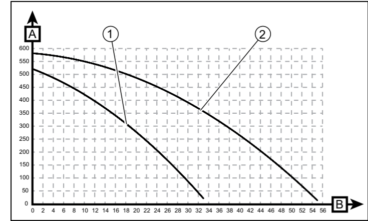
Характеристическая кривая циркуляционного насоса atmoTEC/turboTEC plus VUW
