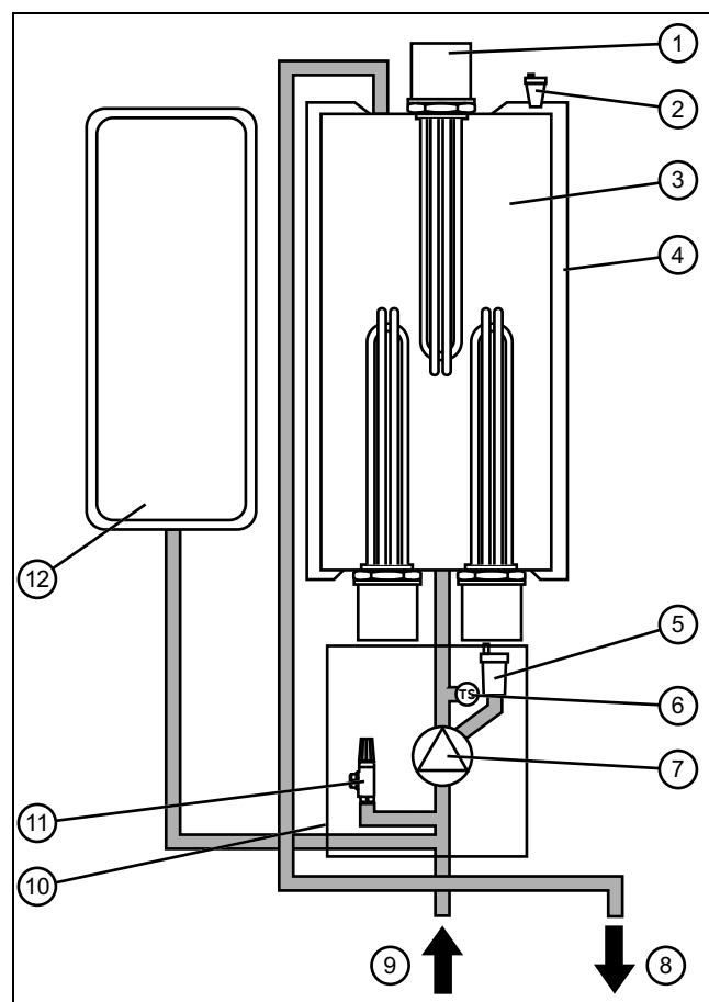
1 Элементы системы отопления 2 Вентиль для выпуска воздуха 3 Ёмкостный водонагреватель / теплообменник 4 Изоляция 5 Автоматический быстродействующий воздухоотводчик 6 Датчик давления 7 Насос системы отопления 8 Подающая линия системы отопления 9 Обратная линия системы отопления 10 Гидравлический узел 11 Предохранительный клапан 12 Расширительный бак
