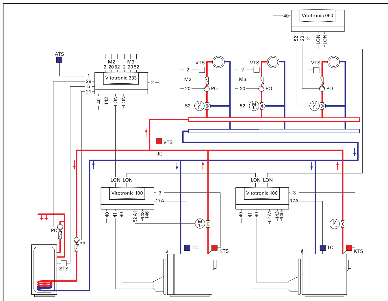
Рис. 3.6. Пример применения: многокотловая установка с регуляторами Vitotronic 100.
