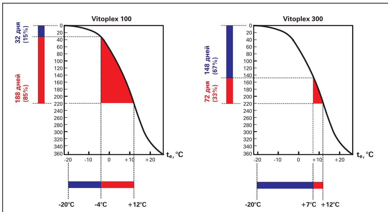
Рис. 13.8. Кривая годового хода температуры наружного воздуха.
