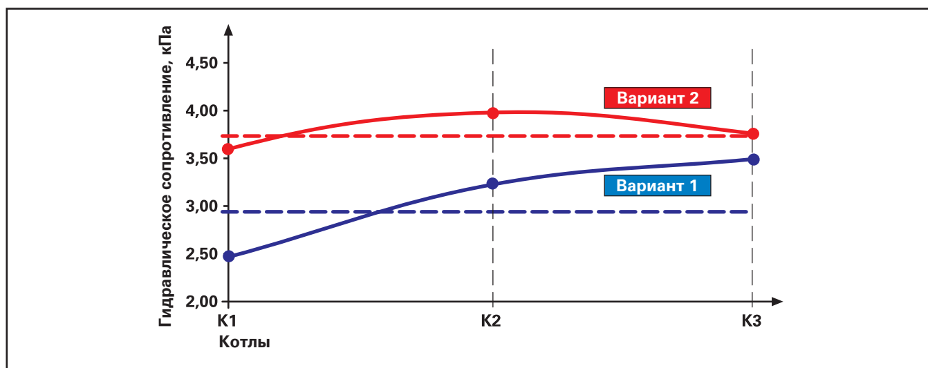
Рис. 13.3. Гидравлическое сопротивление контуров котлов для двух вариантов трубной обвязки
