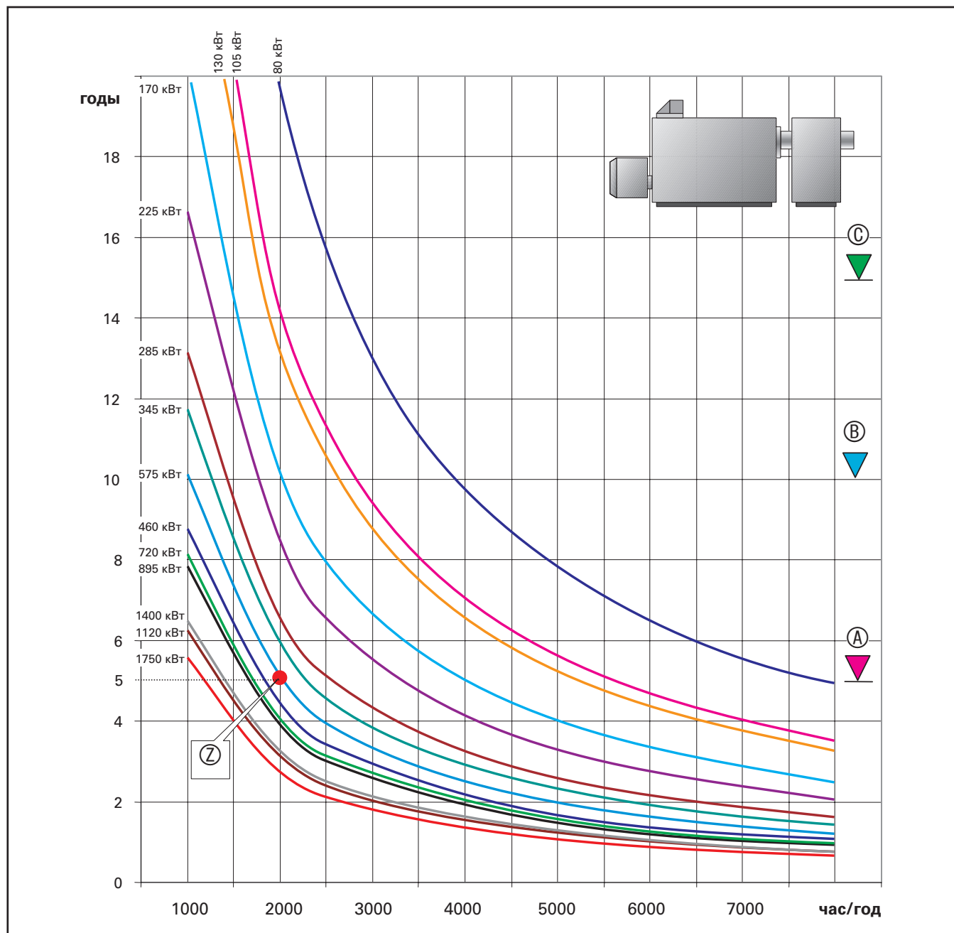
Рис. 8.10. Период окупаемости экономайзера Vitotrans 333 в зависимости от продолжительности его работы с номинальными параметрами в течение года; топливо – природный газ
