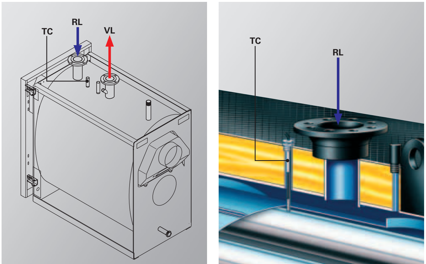
Рис. 3.3. Место установки датчика TC системы Therm-Control в котлах Vitoplex 100, 80-460 кВт, и Vitoplex 300, 80-1750 кВт
