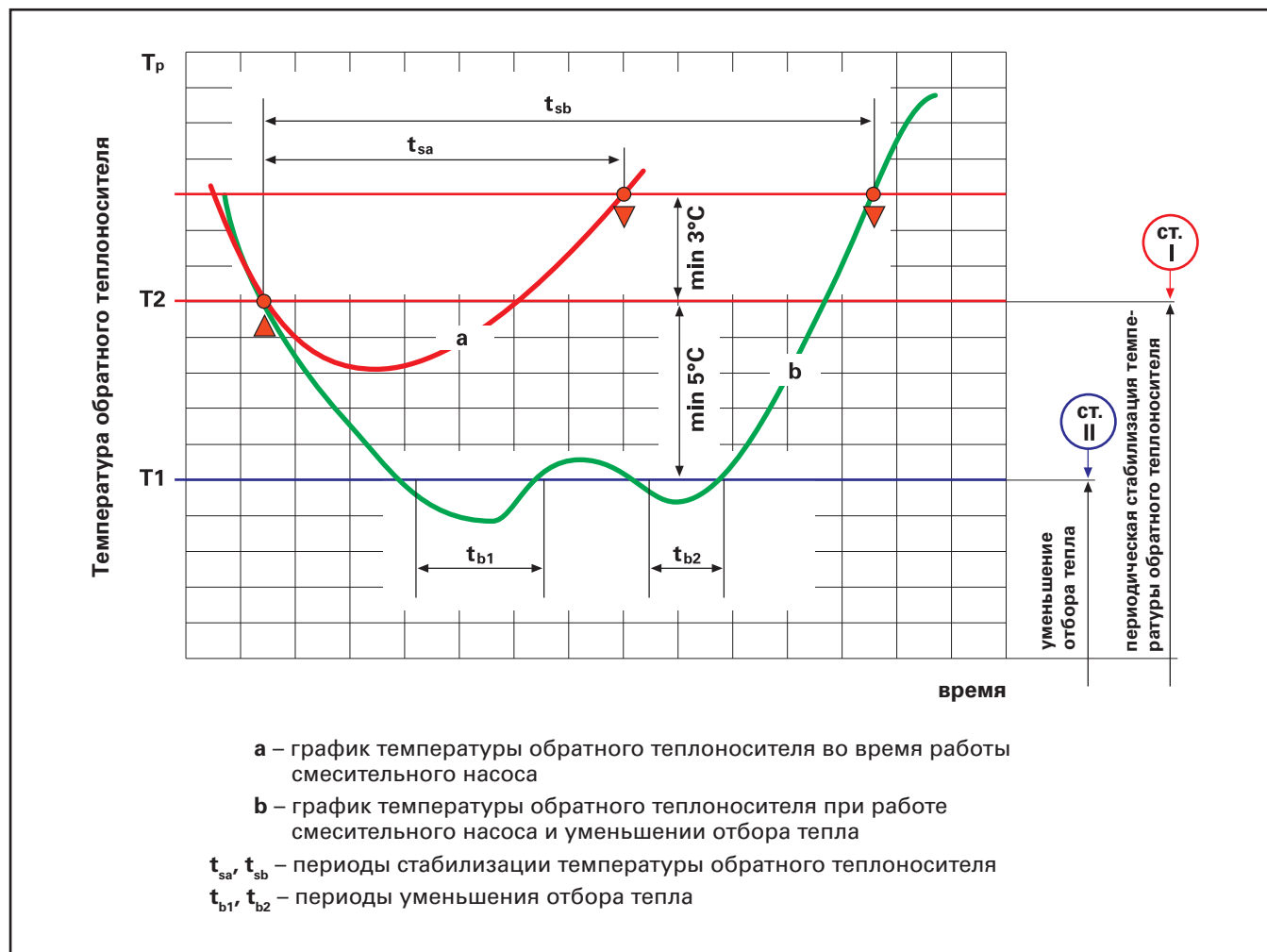
Рис. 3.10. Двухступенчатая система защиты по температуре обратного теплоносителя с использованием смесительного насоса РМ, – класс C2
