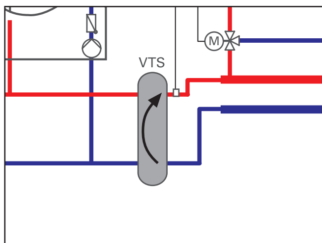
Рис. 8.5. Движение теплоносителя в гидравлической стрелке при работе с конденсационными котлами
