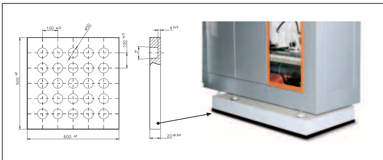
Рис. 14.12. Виброизоляционная плита ADPATA и пример ее применения для блочных ТЭЦ Vitobloc
