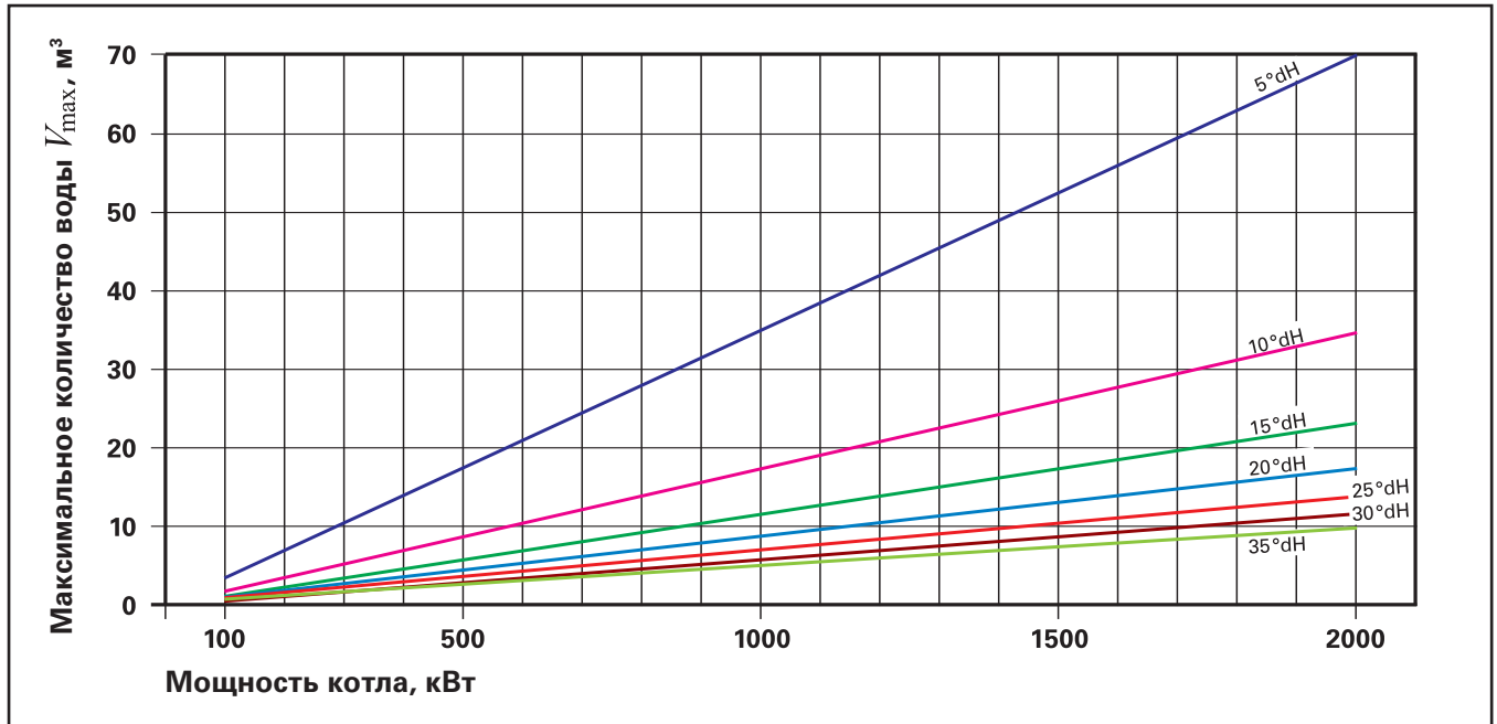
Рис. 15.1. Диаграмма для определения максимального количества воды V_{max} для заполнения и подпитки систем мощностью 100-2000 кВт
