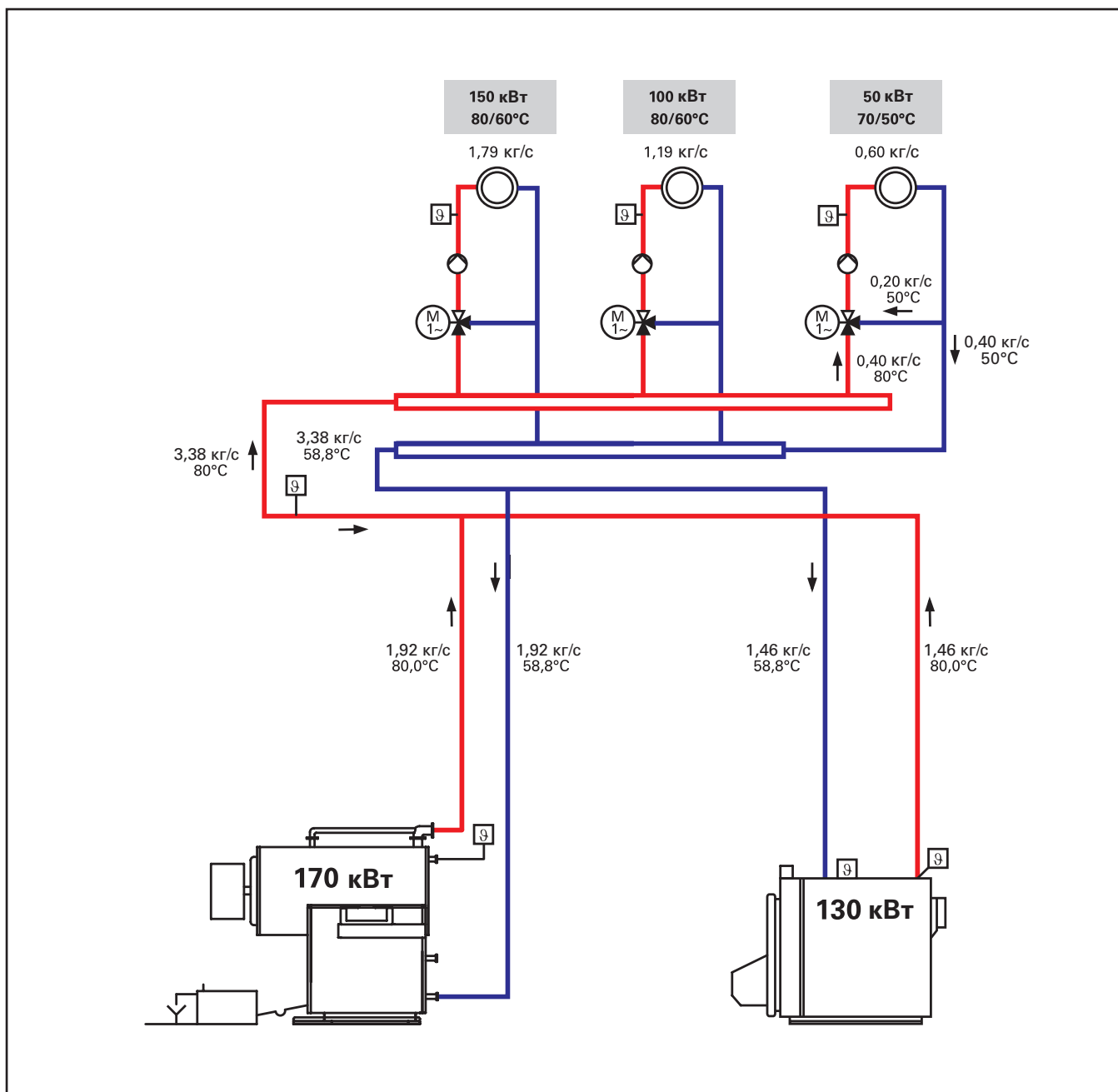
Рис. 8.7. Параллельная каскадная схема котельной с конденсационным котлом Vitocrossal 300 мощностью 170 кВт и низкотемпературным котлом Vitoplex 300 мощностью 130 кВт
