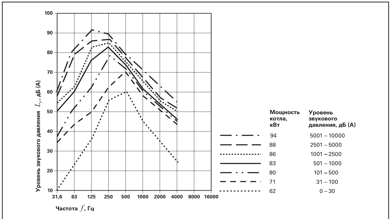
Рис. 14.4. Распределение уровня звукового давления по октавным полосам для группы “котел – вентиляторная горелка” различной мощности
