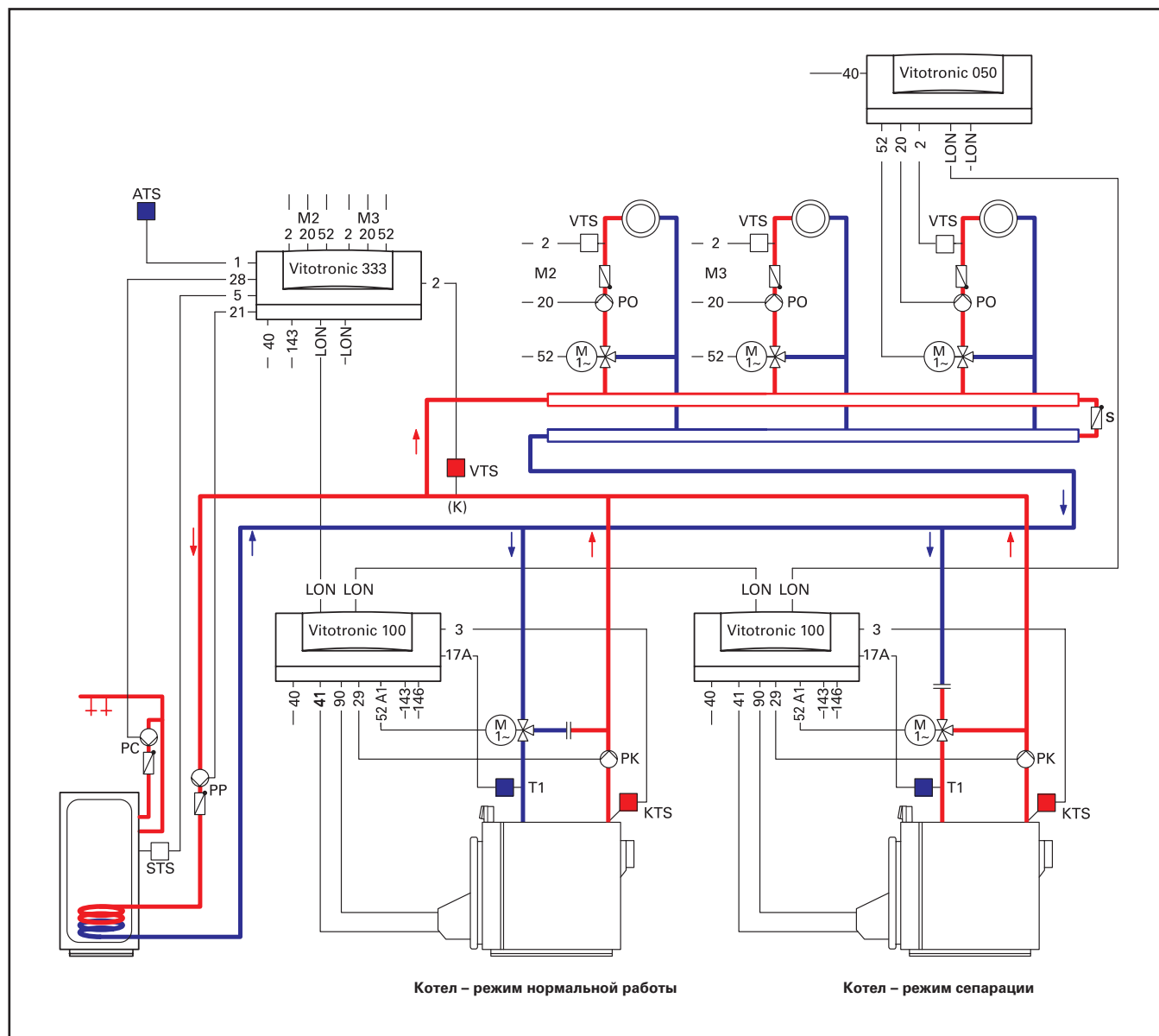
Рис. 3.18. Пример применения: многокотловая установка с регуляторами Vitotronic 100.
