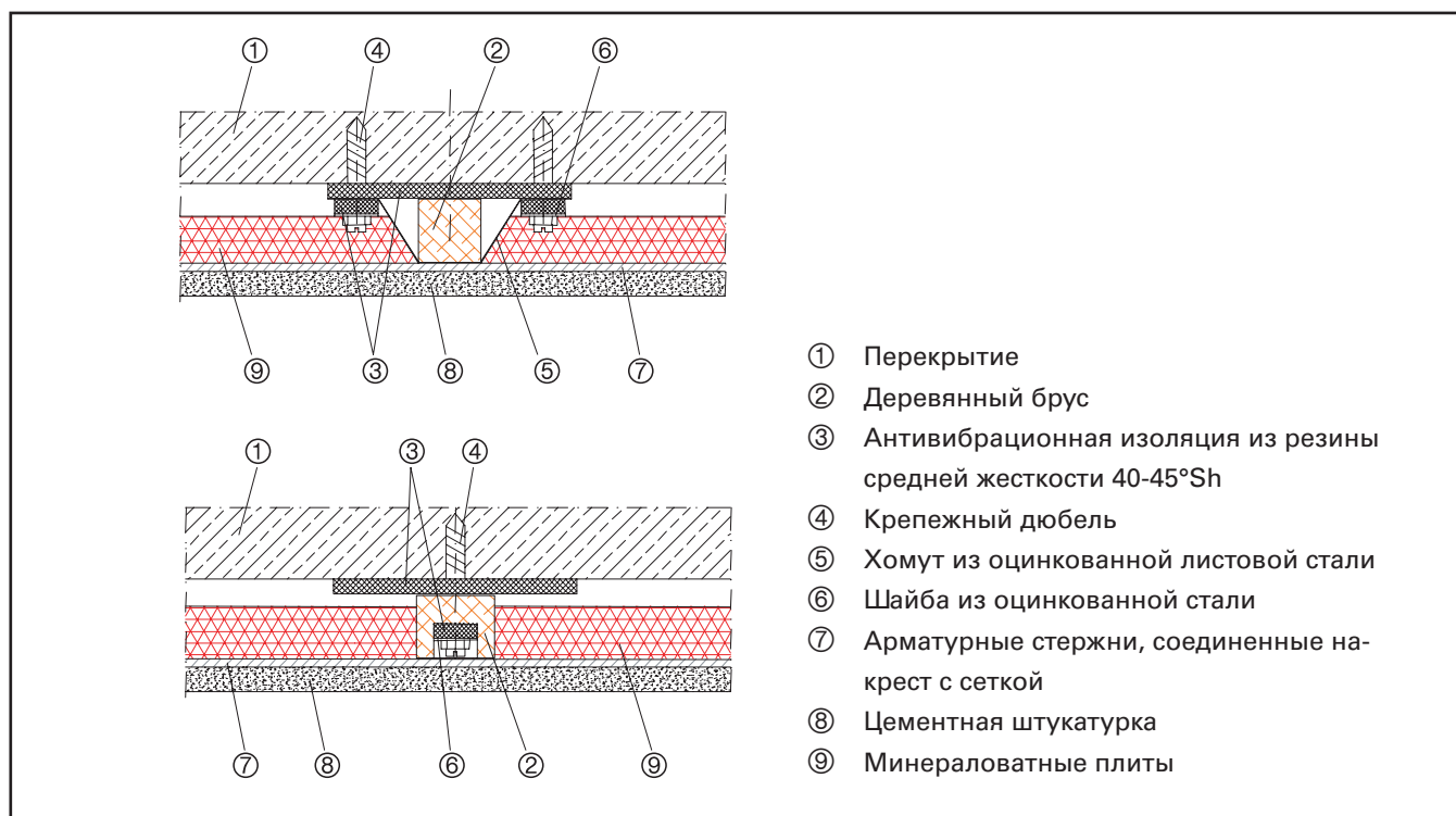
Рис. 14.19. Примеры конструкции подвесных потолков
