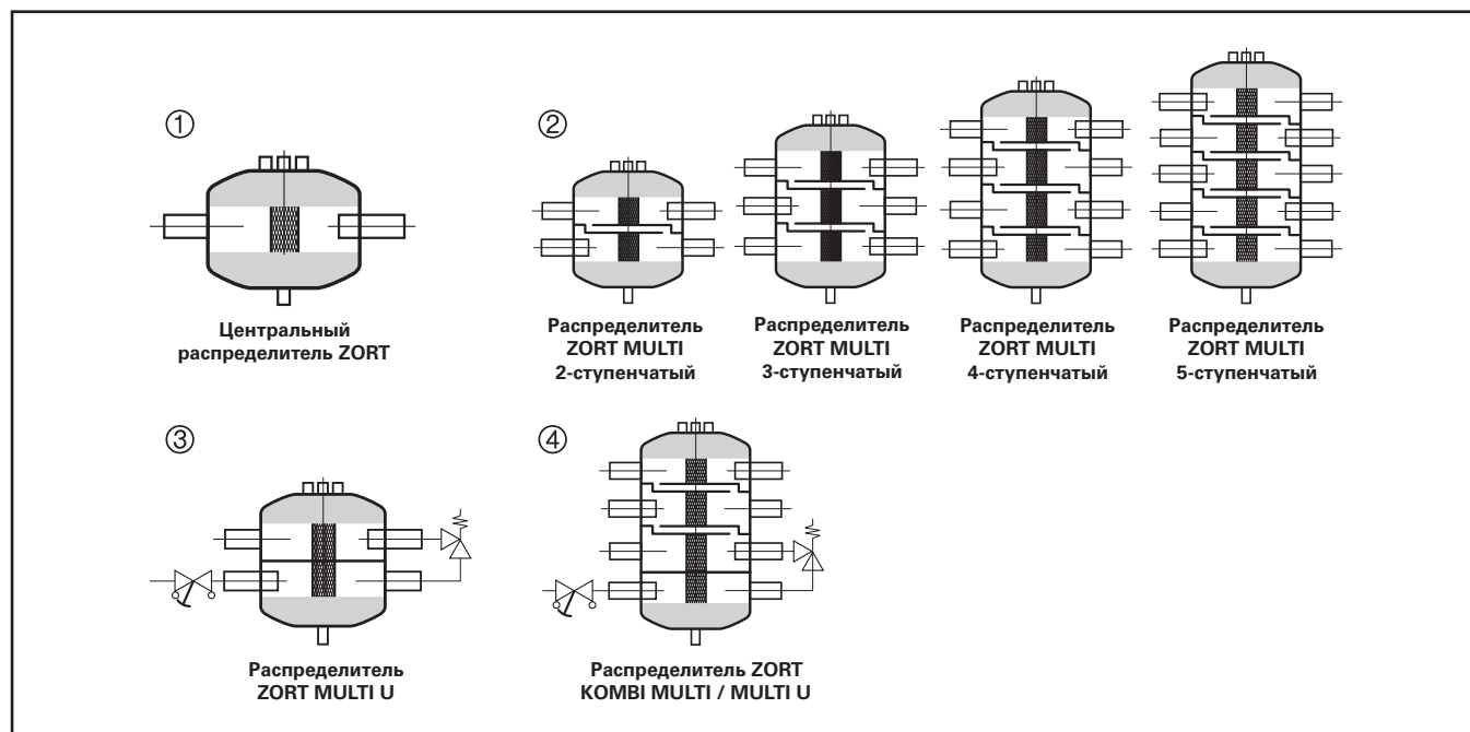
Рис. 3.22. Гидравлические распределители
