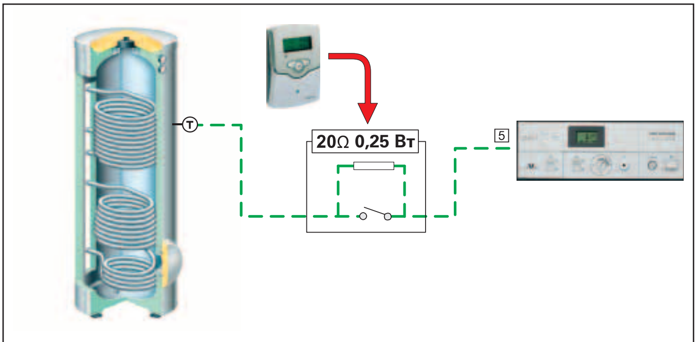
Рис. 12.3. Совместная работа регулятора Vitosolic 100/200 с регулятором котла, не оснащенным коммуникационной шиной KM-BUS. Включение дополнительного сопротивления в цепь датчика температуры воды в бойлере ГВС
