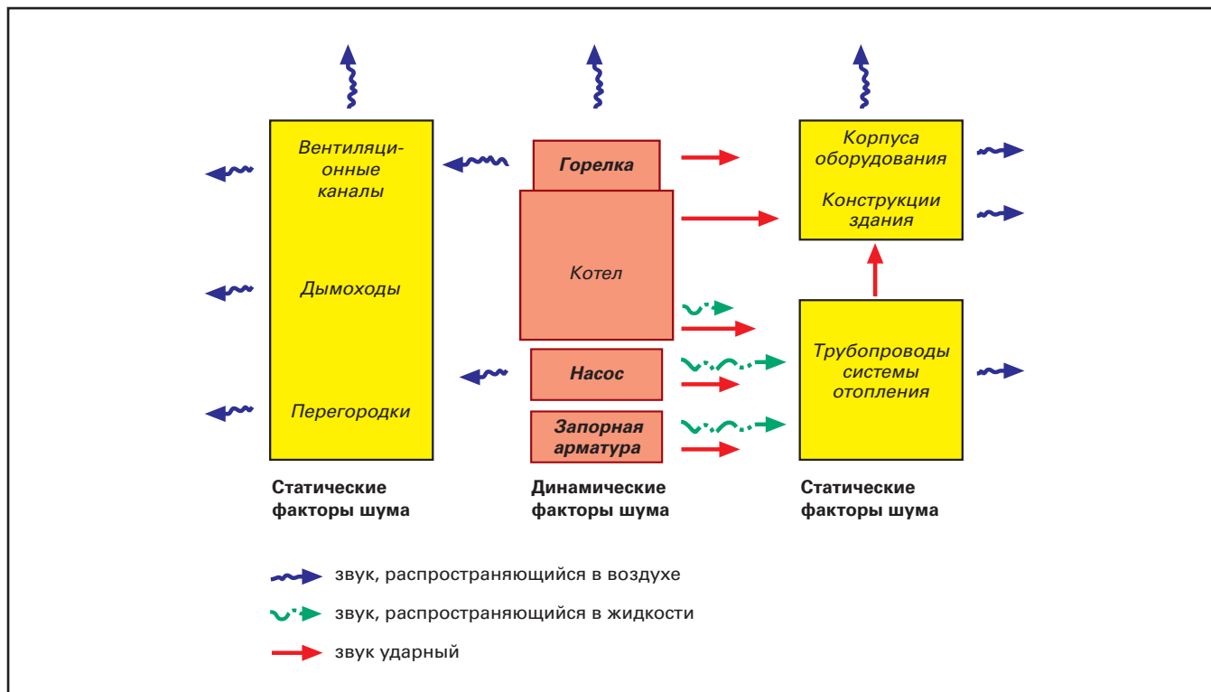
Рис. 14.8. Акустическая модель котельной и системы отопления
