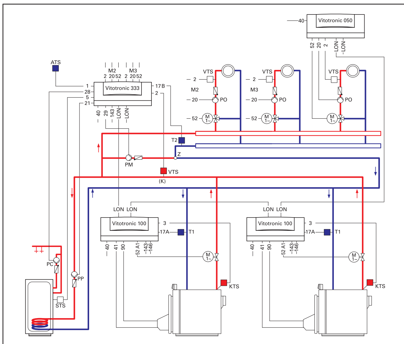
Рис. 3.8. Пример применения: многокотловая установка с регуляторами Vitotronic 100.
