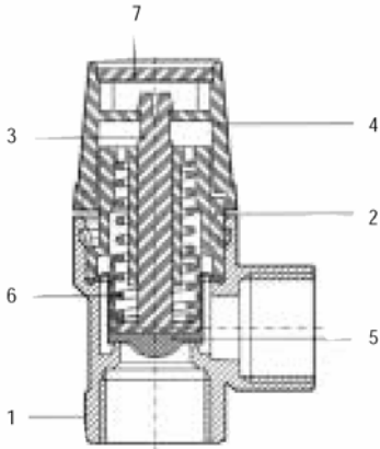
1.Корпус. 2. Крышка корпуса. 3. Тяга мембраны. 4, 5 Поворотная мембрана. 6. Пружина. 7 Табличка с обозначением.
